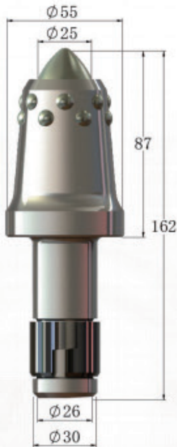
GL87 30-U84 Z2535E14-C-加强(RS1)
